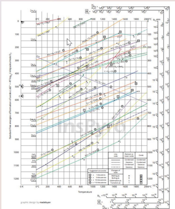
شکل 4: دیاگرام الینگهام هیدروژن
