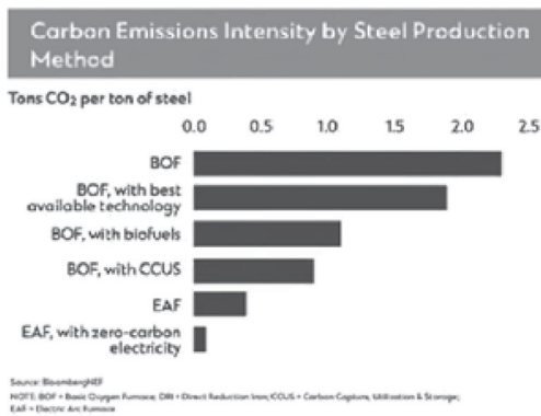
شکل ۱: شدت انتشار کربن در روش‌های مختلف تولید فولاد
